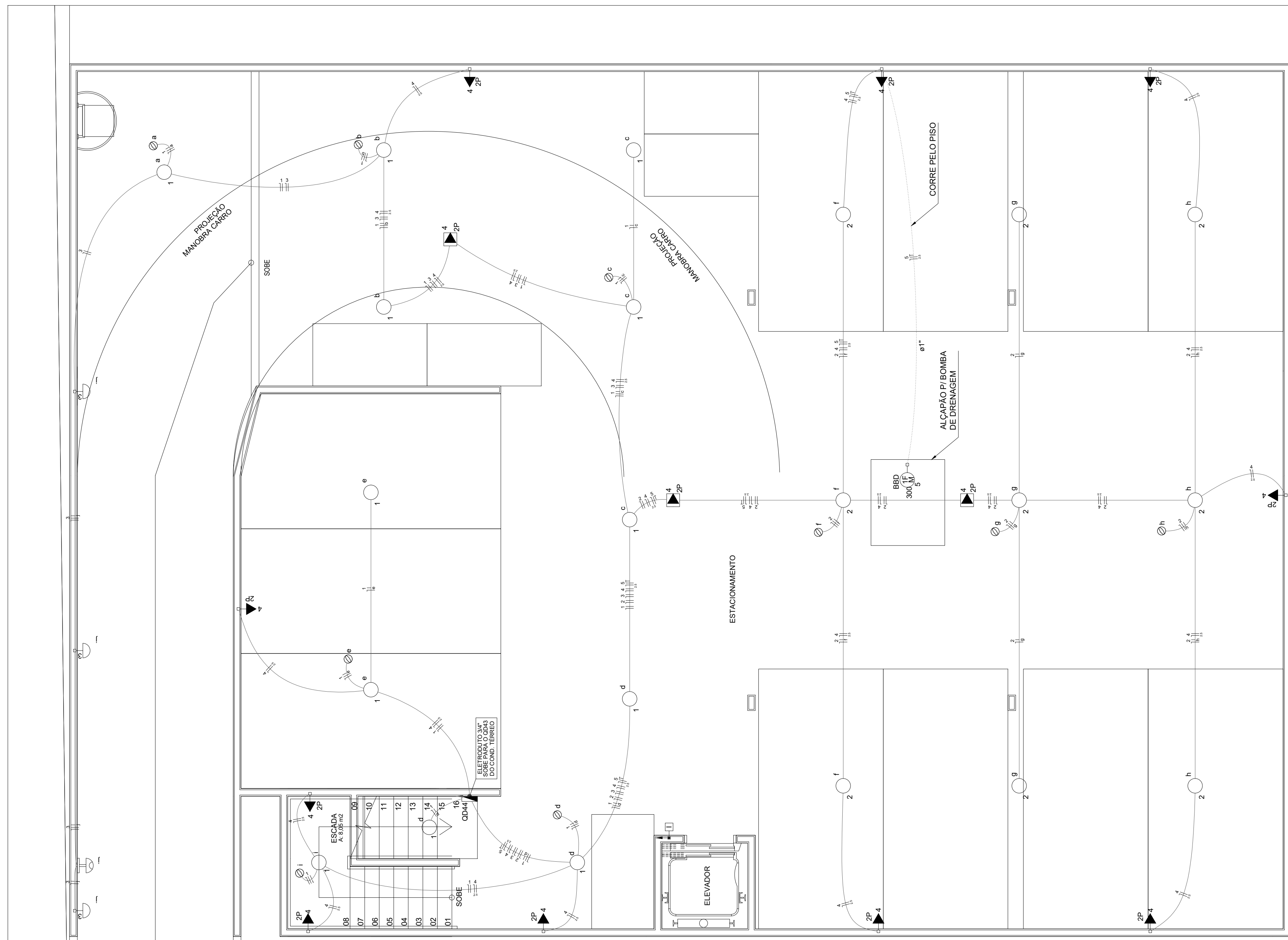
1 PLANTA BAIXA DO PAVIMENTO SUBSOLO 2 ESCALA 1:50
