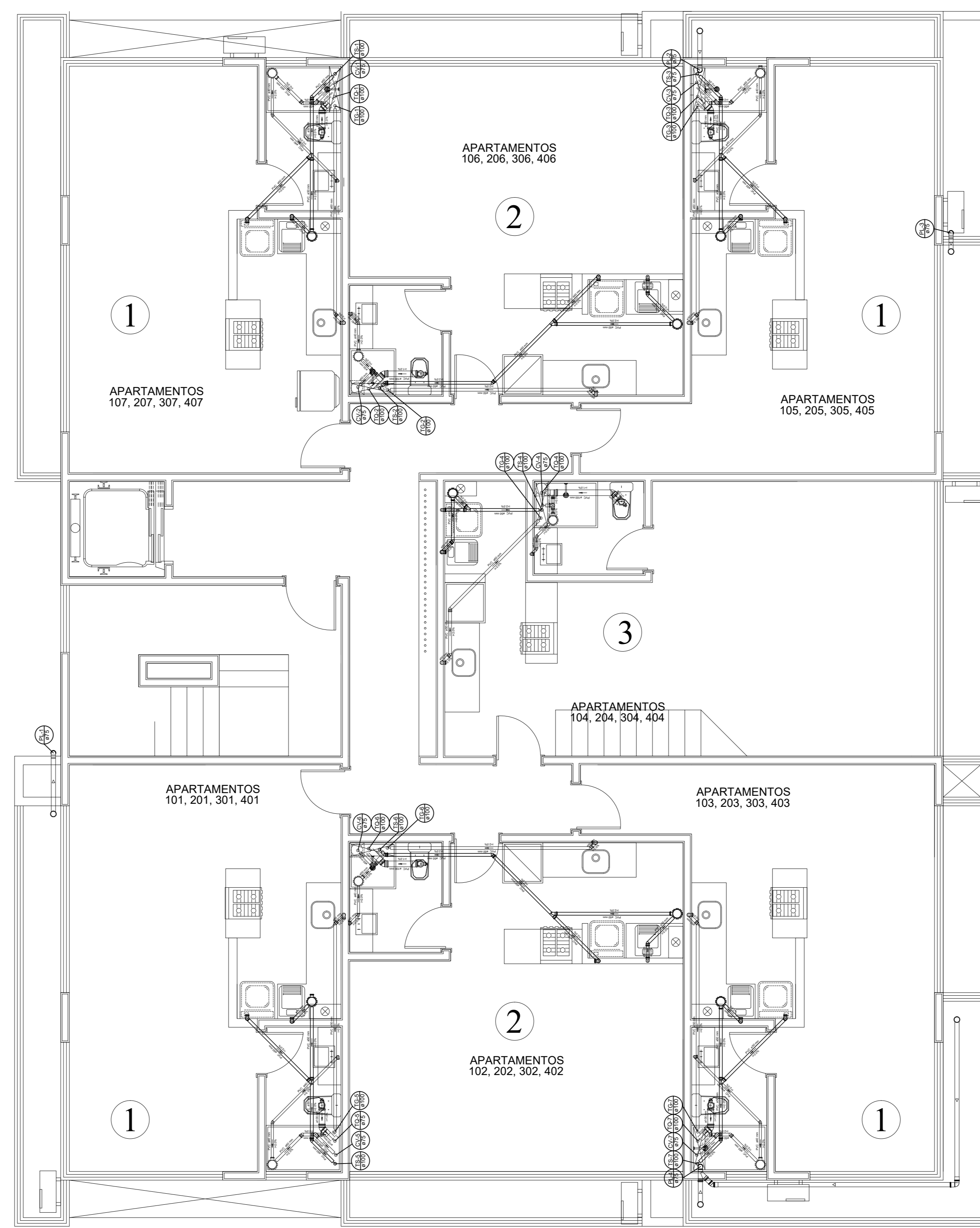
2 PLANTA BAIXA PAV. TIPO - REDE DE ESGOTO ESCALA 1:50
