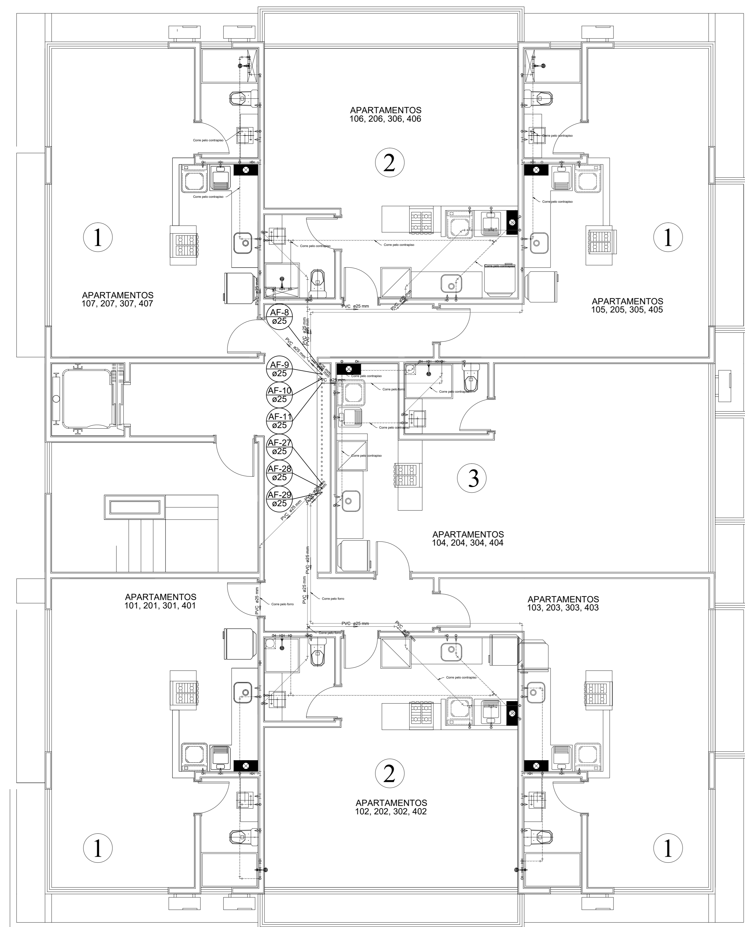
1 PLANTA BAIXA PAV. TIPO - REDE DE ÁGUA ESCALA 1:50
