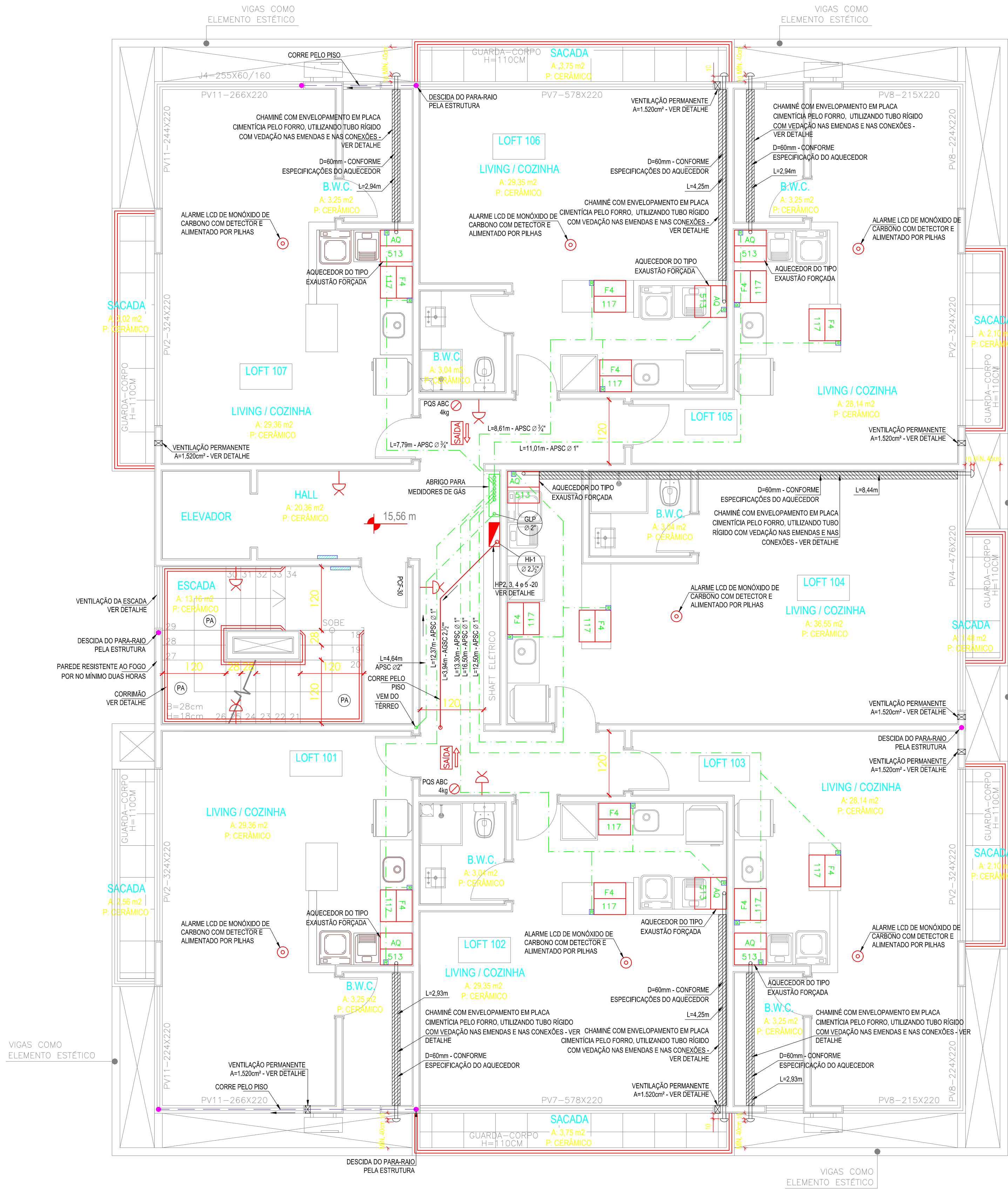
1 PLANTA BAIXA PVTO TIPO 1 ESCALA 1:50
